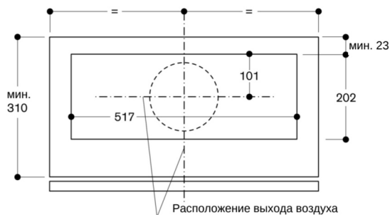
Вид шкафа сверху с AC 200 и AA 211 812
