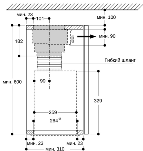
Разрез навесного шкафа с AC 200 и AA 211 812
